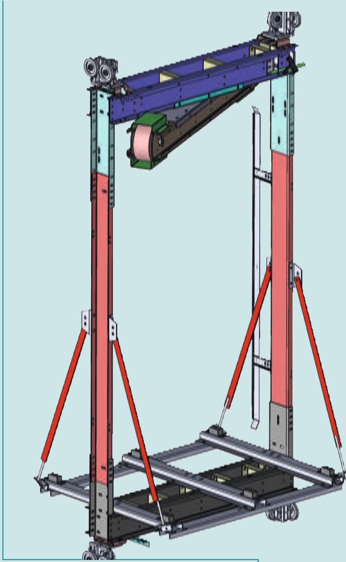
Cabin Frame Structure De Cabine КАРКАС КАБИНЫ شريحة الكابينة
