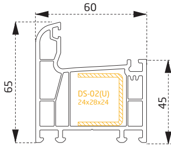
PRVNEC01B Kasa Profili Frame Profile
