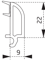
PSC9660BY 40 mm Cam Çıtası 40 mm Glazing Bead
