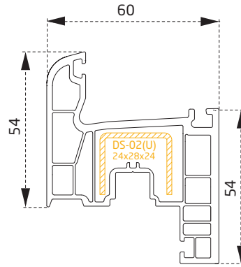
PRVNEC02B Kanat Profili Sash Profile
