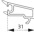
PFS1460BY Tek Cam Çıtası Single Glazing Bead
