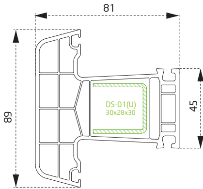
PDR0360BY Orta Kayıt Profili Mullion Profile
