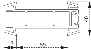
PEX2560BY Geniş Bağ Profili Wide Band Profile
