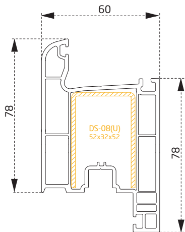
PRVNEC04B Kapi Profili Opening Door Profile
