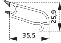
PVN1460BY Tek Cam Çıtası Single Glazing Bead
