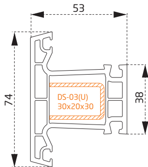
PFS0360BY Orta Kayıt Profili Mullion Profile
