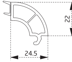
PSC1960BY 24 mm Cam Çıtası 24 mm Glazing Bead
