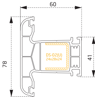
PRVNEC03B Orta Kayıt Profili Mullion Profile
